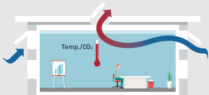
Atriumlüftung
